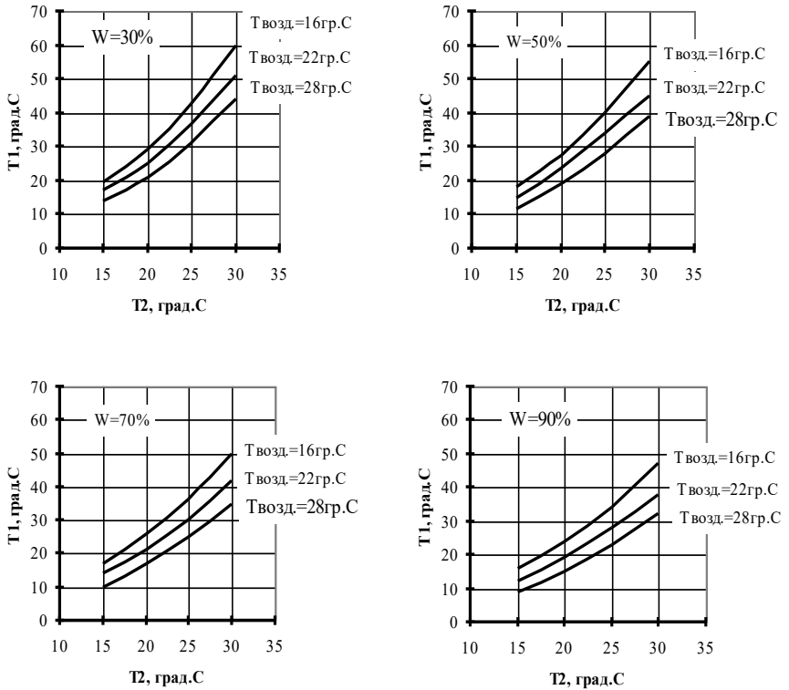
Рис.7. Графики охлаждения при расходе воды 40 м 3 /ч:
