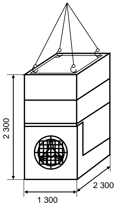
Рис. 5. Схема строповки градирни.
