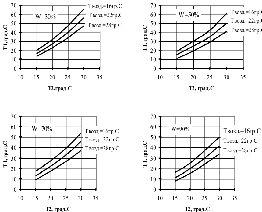
Рис.6. Графики охлаждения при расходе воды 30 м³/ч:
