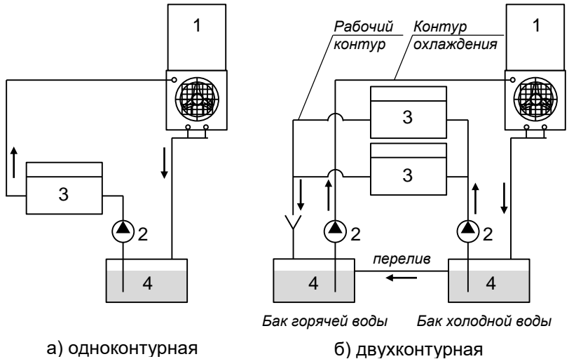
Рис.2. Схемы систем оборотного водоснабжения:
