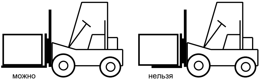
Рис.5. Схема транспортировки корпуса верхнего градирни вилочным погрузчиком.
