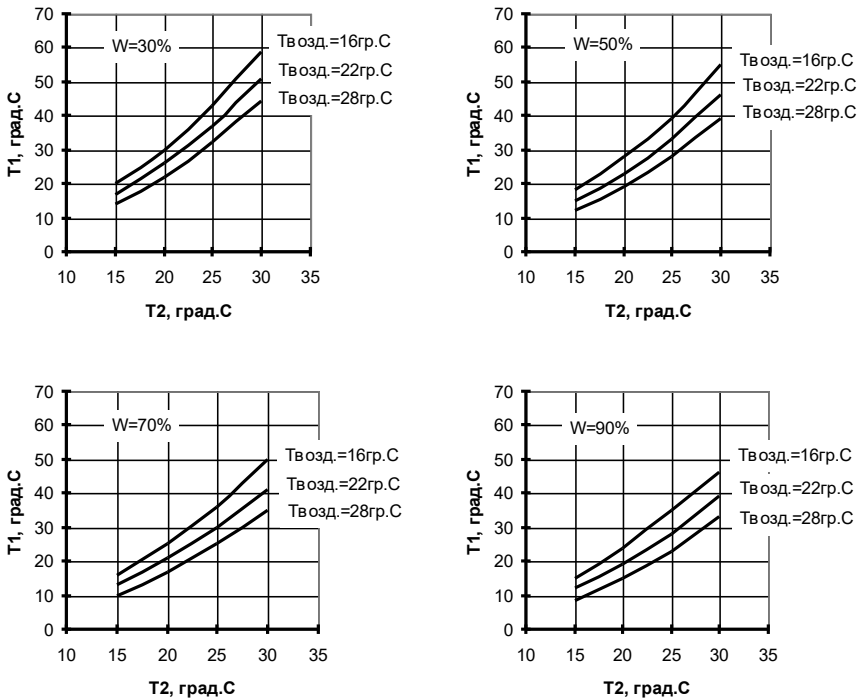
Рис.6. Графики охлаждения при расходе воды 50 м 3 /ч:
