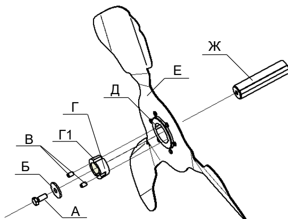
Рис.3. Рабочее колесо вентилятора.
