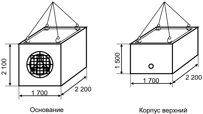
Рис.4. Схема строповки градирни.
