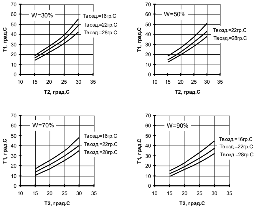
Рис.7. Графики охлаждения при расходе воды 60 м 3 /ч:
