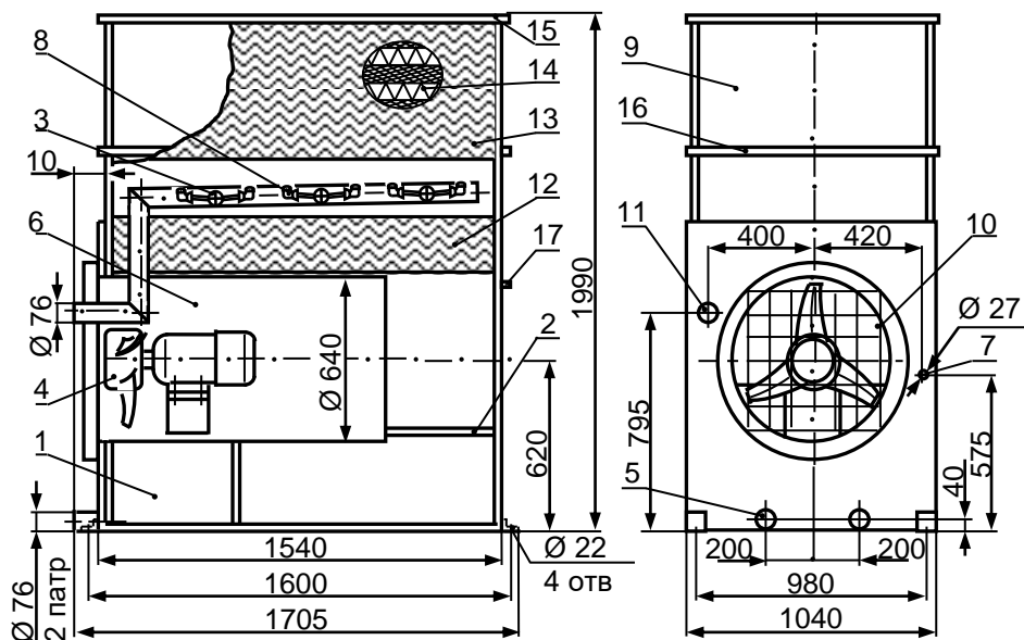
Рис. 1. Схема градирни
