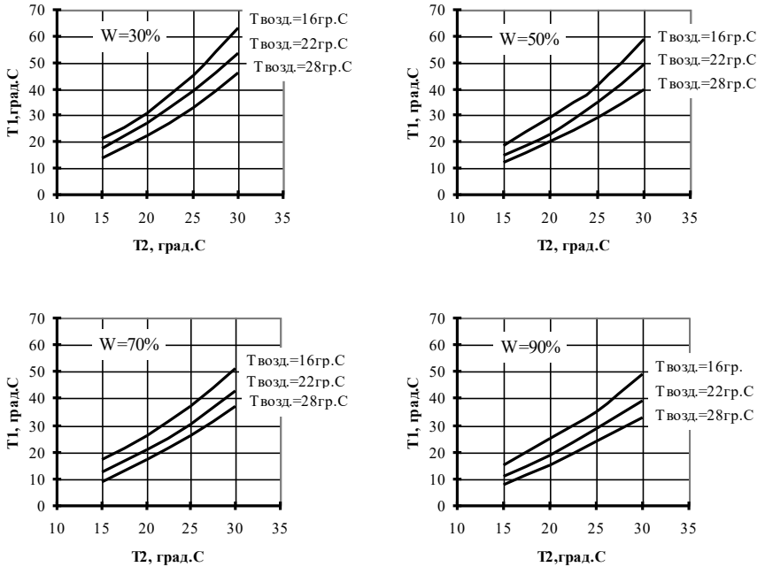
Рис.7. Графики охлаждения при расходе воды 20 м 3 /ч:
