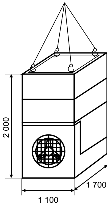
Рис.5. Схема строповки градирни.
