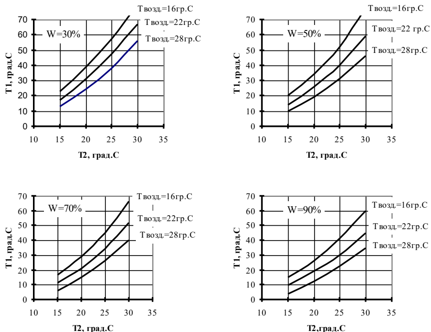
Рис.6. Графики охлаждения при расходе воды 10 м 3 /ч:
