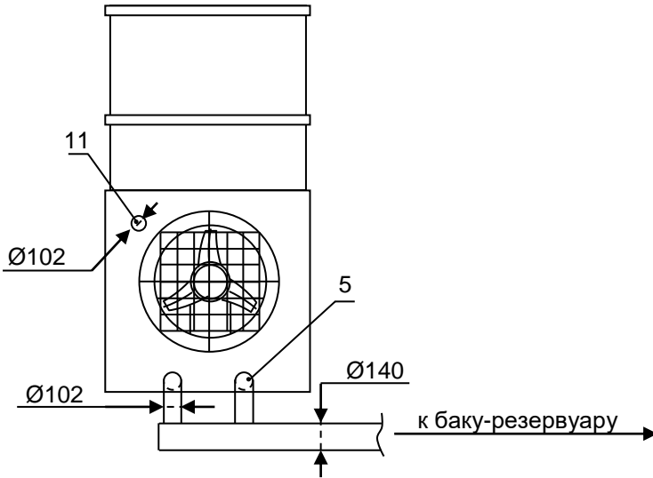
Рис.3. Схема подвода сливной магистрали.
