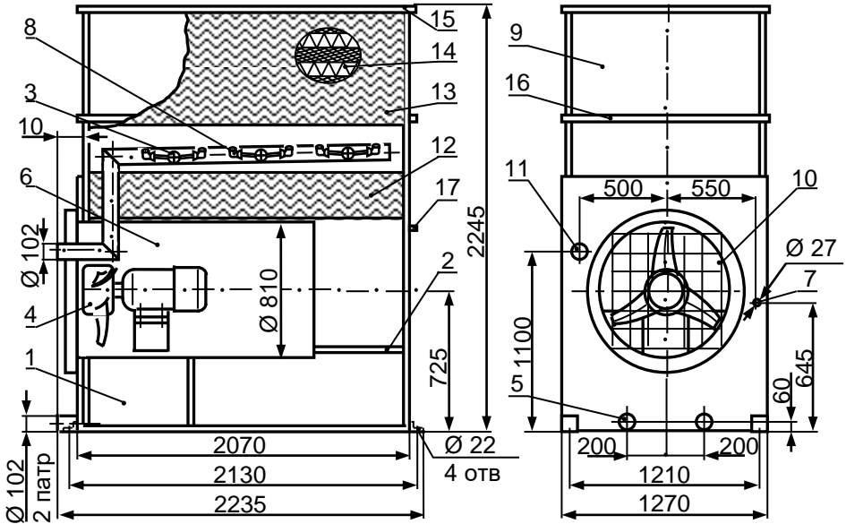
Рис. 1. Схема градирни
