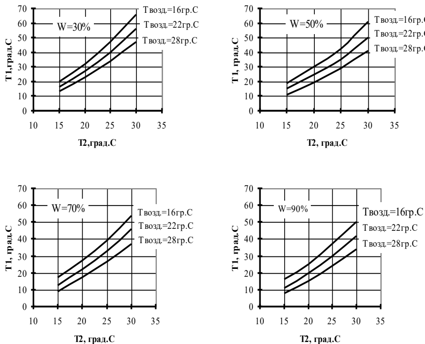
Рис.6. Графики охлаждения при расходе воды 30 м 3 /ч:
