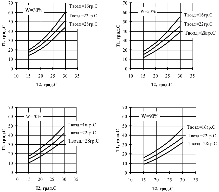
Рис.7. Графики охлаждения при расходе воды 40 м³/ч:
