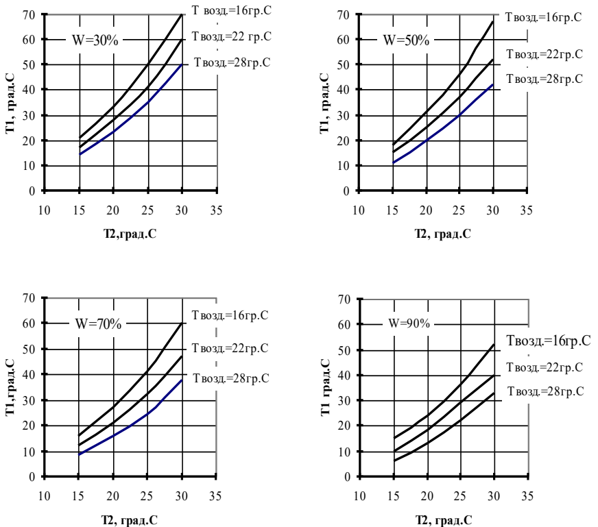
Рис.6. Графики охлаждения при расходе воды 5 м 3 /ч:
