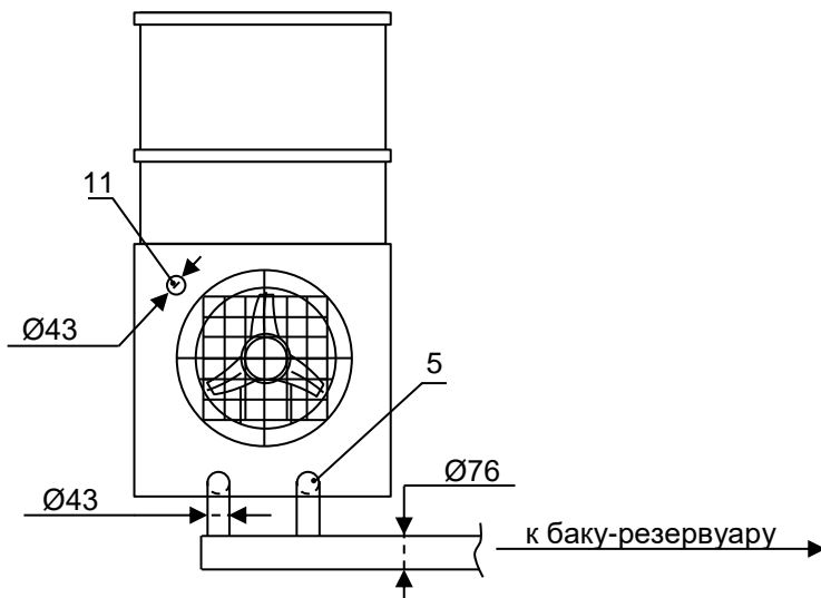
Рис.3. Схема подвода сливной магистрали.
