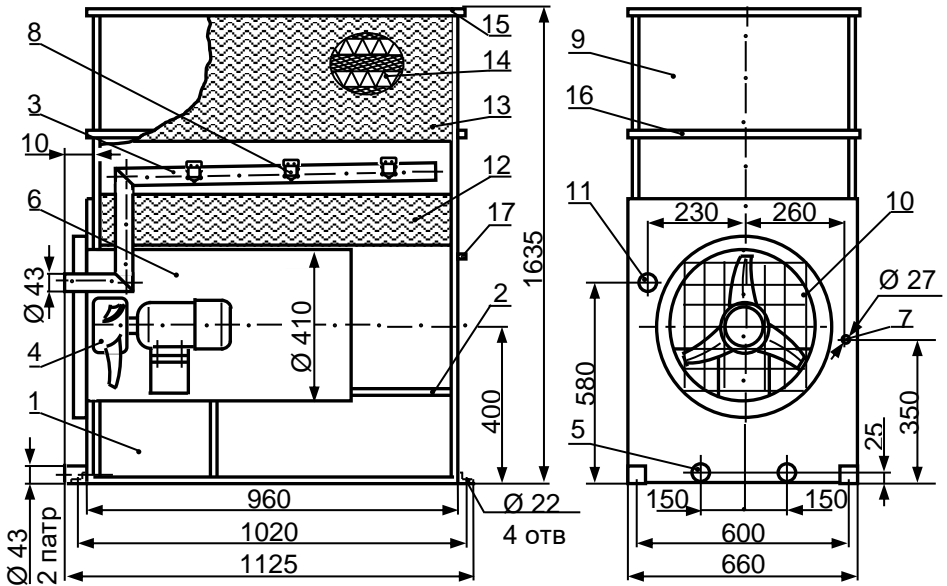
Рис. 1. Схема градирни
