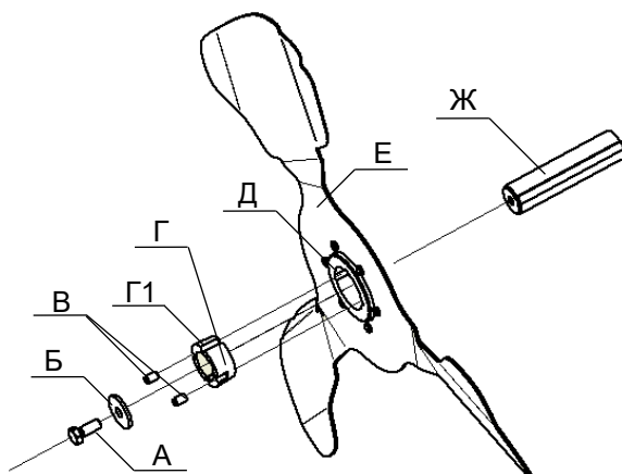
Рис.4. Рабочее колесо вентилятора.
