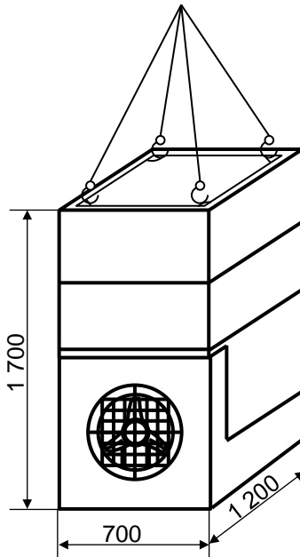
Рис.5. Схема строповки градирни.
